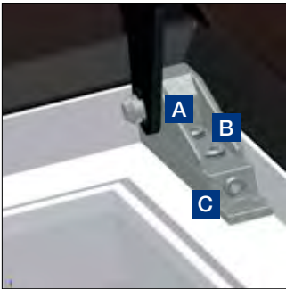
Regulacja wysokości położenia skrzydła w ościeżnicy A, B - wkręty zaciskowe C - wkręt regulacji
