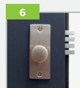
Zamek dodatkowy górny 4-ryglowy z wkładko- gałką (system jednego klucza)
