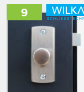
Zamek dodatkowy górny z wkładką-gałką WILKA® (system jednego klucza)
