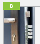
Zamek główny 4-ryglowy z wkładką (system jednego klucza)
