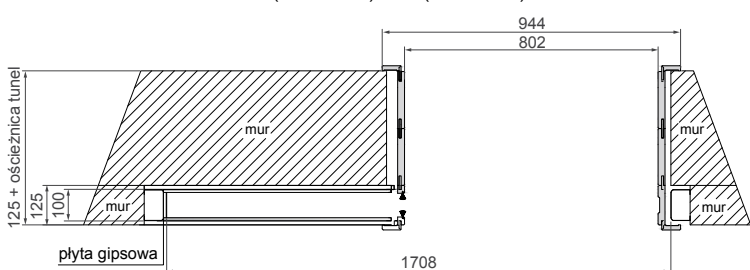
OŚCIEŻNICA ZAKRES (200-220) DO (400-420) – ASYMETRYCZNA
