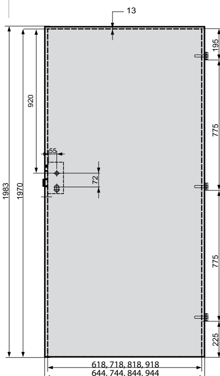
SKRZYDŁO PRZYLGOWE W NORMIE CZESKIEJ
