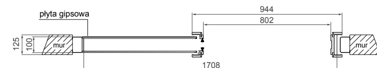
OŚCIEŻNICA ZAKRES (126-200) – SYMETRYCZNA*
