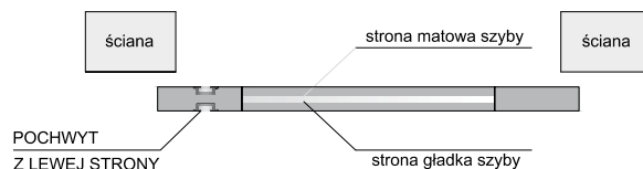
SKRZYDŁO PRAWE BEZFELCOWE (PRZESUWANE W PRAWO)
