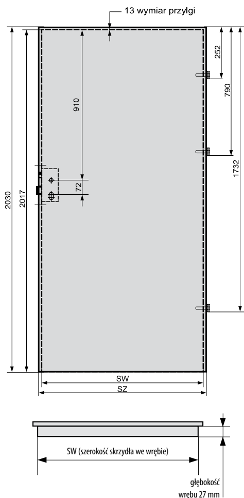
SKRZYDŁO PRZYLGOWE W NORMIE CZESKIEJ
