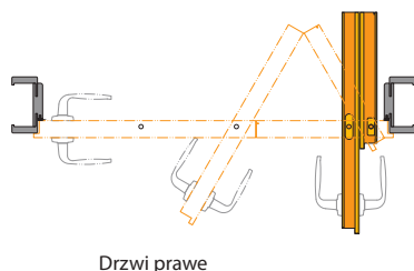
SPOSÓB OTWIERANIA DRZWI* (rzut z góry)
