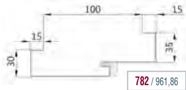
Ościeżnica metalowa do drzwi RC3
