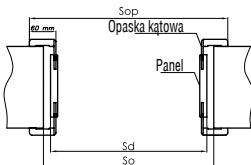
Tunel ZT z opaskami OK6
