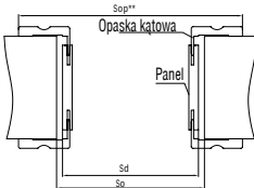
Tunel ZT z opaskami Q-SYSTEM
