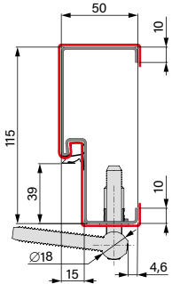
OŚCIEŻNICA STALOWA
