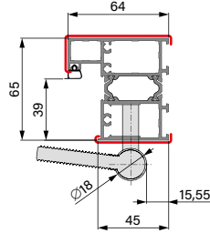
OŚCIEŻNICA ALUMINIOWA
