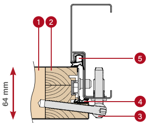
OŚCIEŻNICA STALOWA
