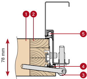
OŚCIEŻNICA STALOWA
