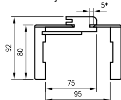
Przekrój ORB 075
