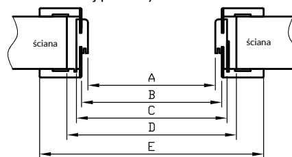
Przekrój poziomy ORB
