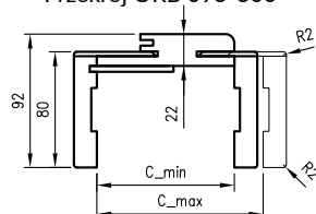
Przekrój ORB 095-300
