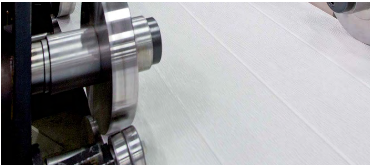
Nowoczesna, sterowana komputerowo linia technologiczna o długości ponad 200 m produkująca w systemie ciągłym panele do bram segmentowych - na zdjęciach jeden z etapów kształtowania blachy.
