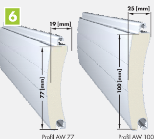
Dwa rodzaje profili
