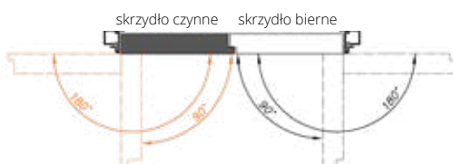
C. Drzwi lewe otwierane na zewnątrz
