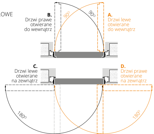
B. Drzwi prawe otwierane do wewnątrz
