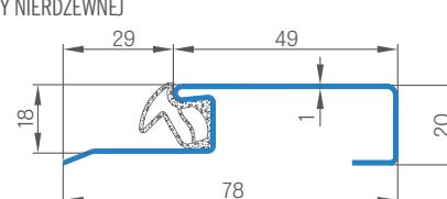
PRÓG Z BLACHY NIERDZEWNEJ
