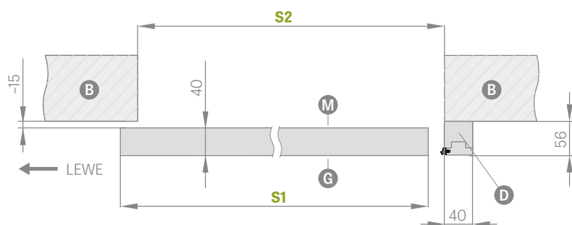
SP2N (wersja rewers)
