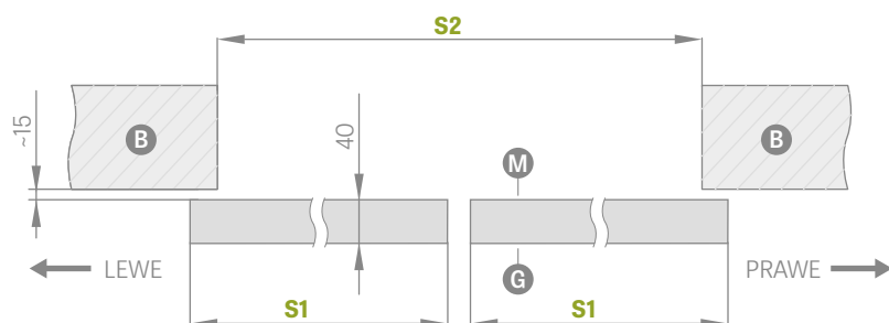
SP2N (wersja rewers)
